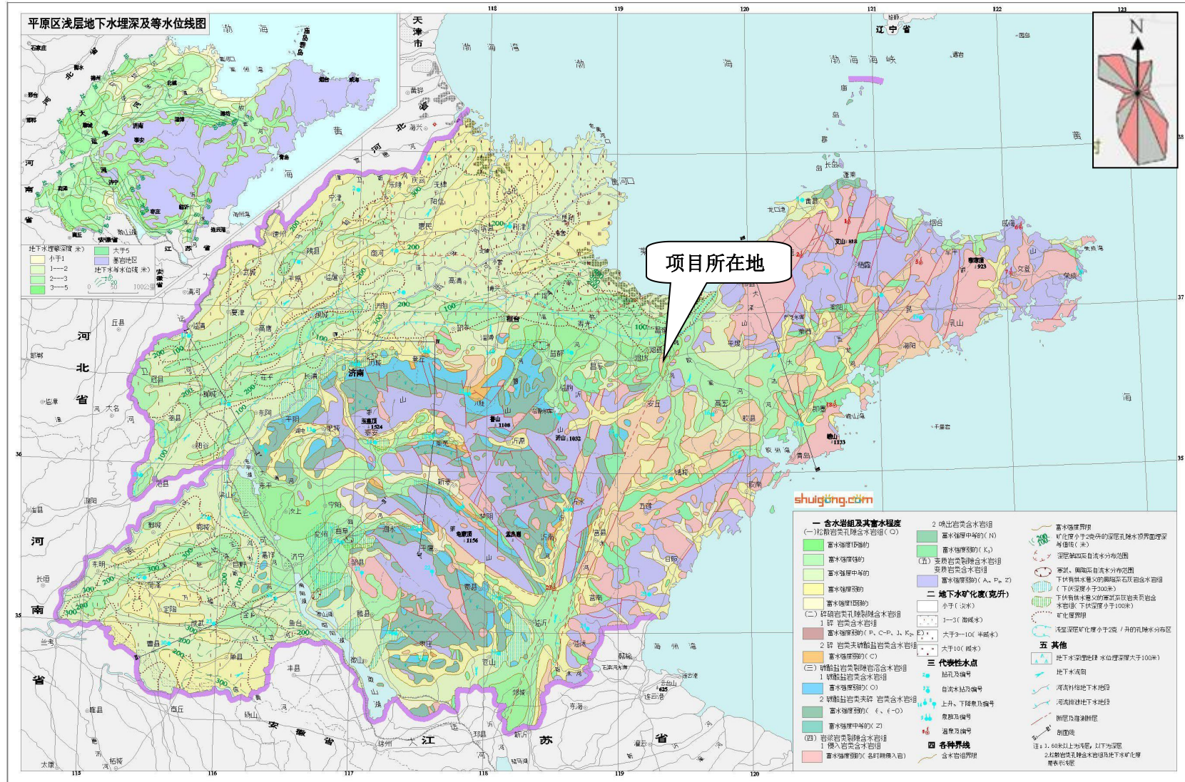
图 3.1-2 项目所在地水文地图 比例尺 1: 3300000
