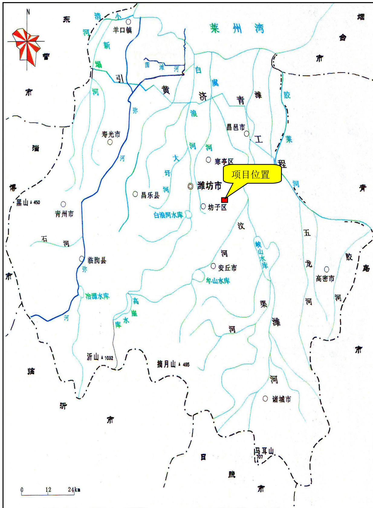
图 3.1-3 项目区地表水系图
